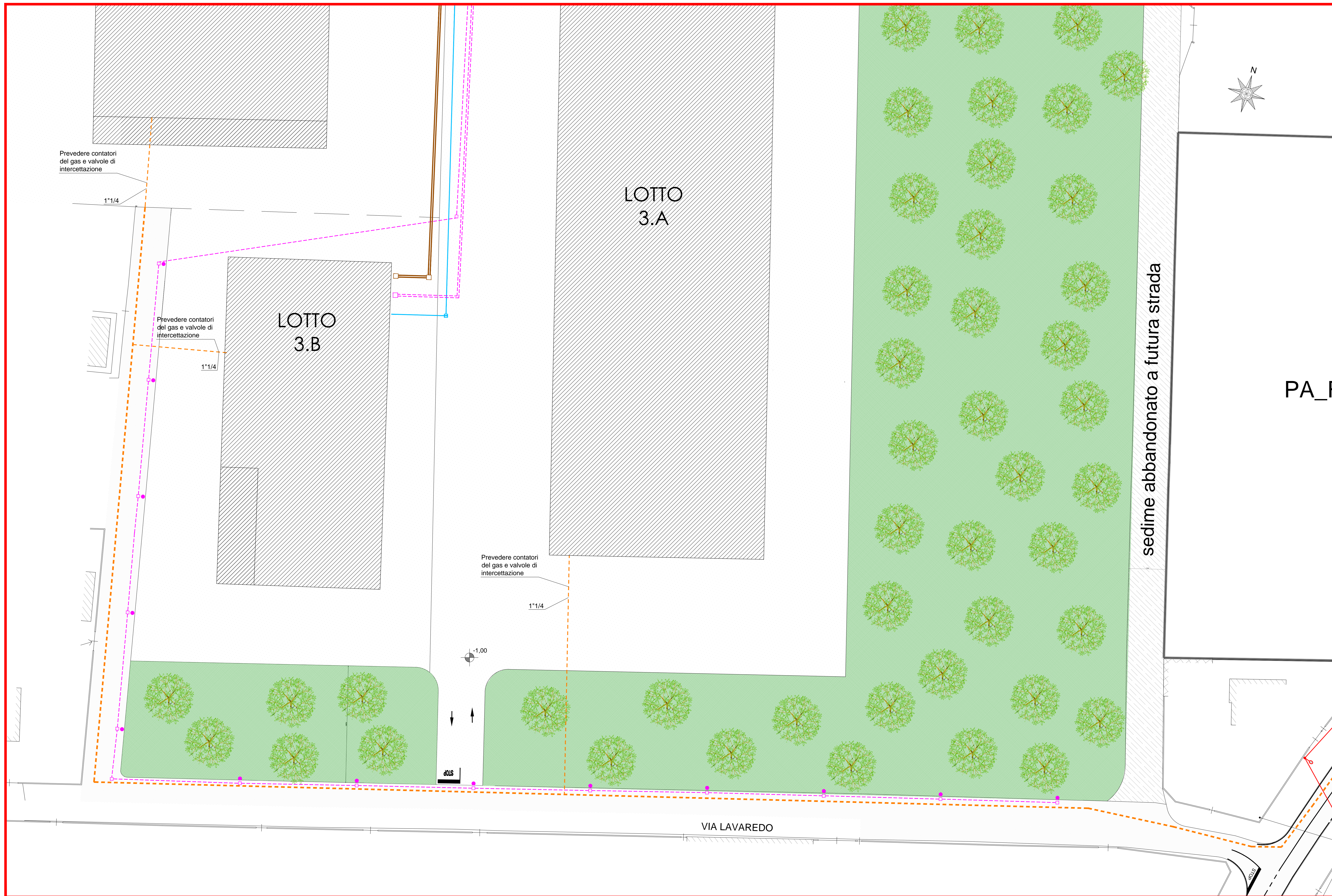
PLANIMETRIA GENERALE DI PROGETTO RETI ENEL-TELECOM-ACQUA-GAS- INQUADRAMENTO 3 - SCALA 1:250
