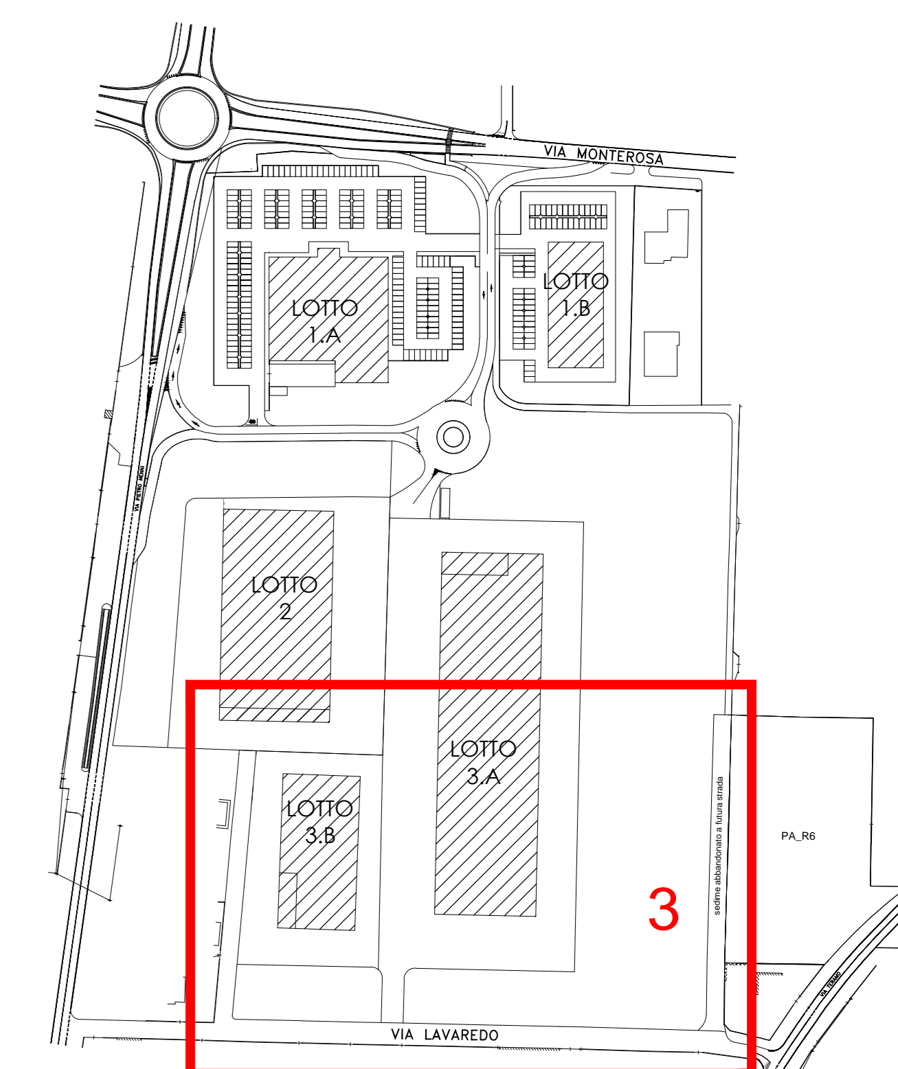
PIANTA CHIAVE - SCALA 1:2000
